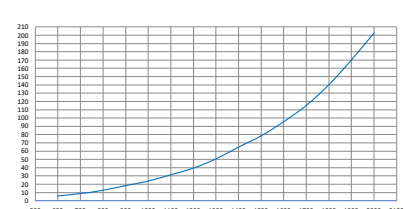
6M33.3 P4 750@2000rpm - BSFC (L/h)
